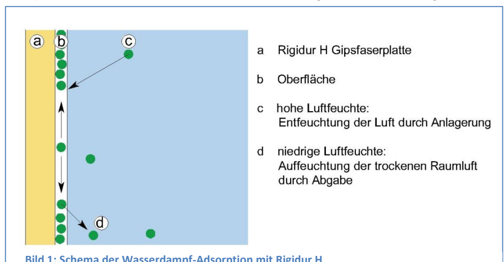
Bild 1: Schema der Wasserdampf-Adsorption mit Rigidur H
